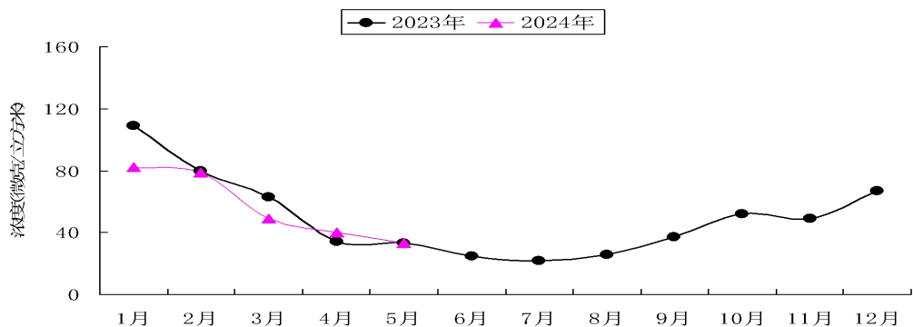
图3 濮阳市环境空气 PM 2.5 月均浓度走势图
