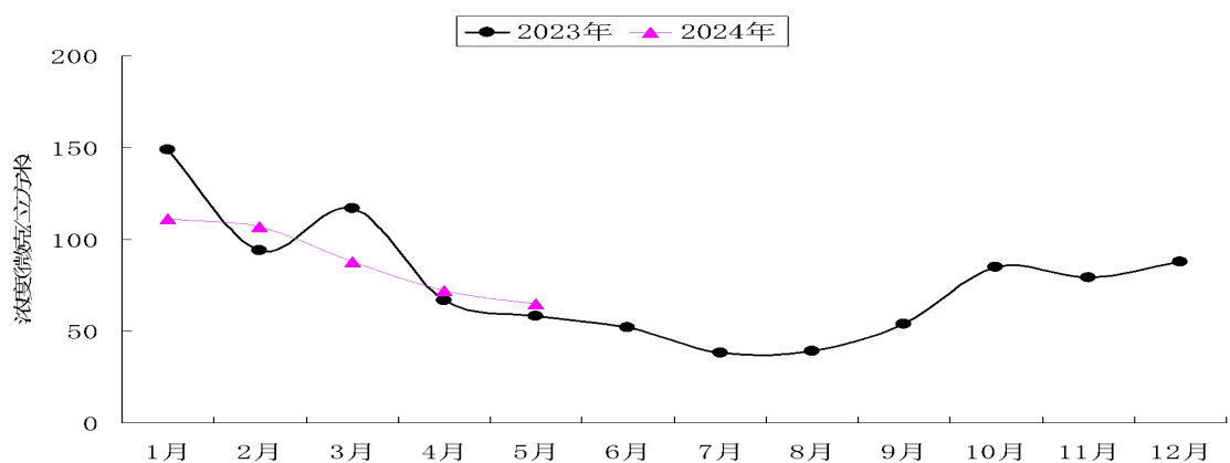
图4 濮阳市环境空气 PM 10 月均浓度走势图
